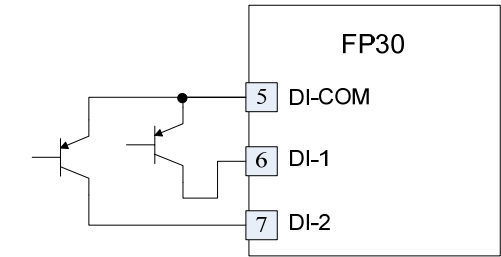
集电极开路接线示意图
