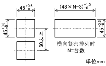
面板开口图
